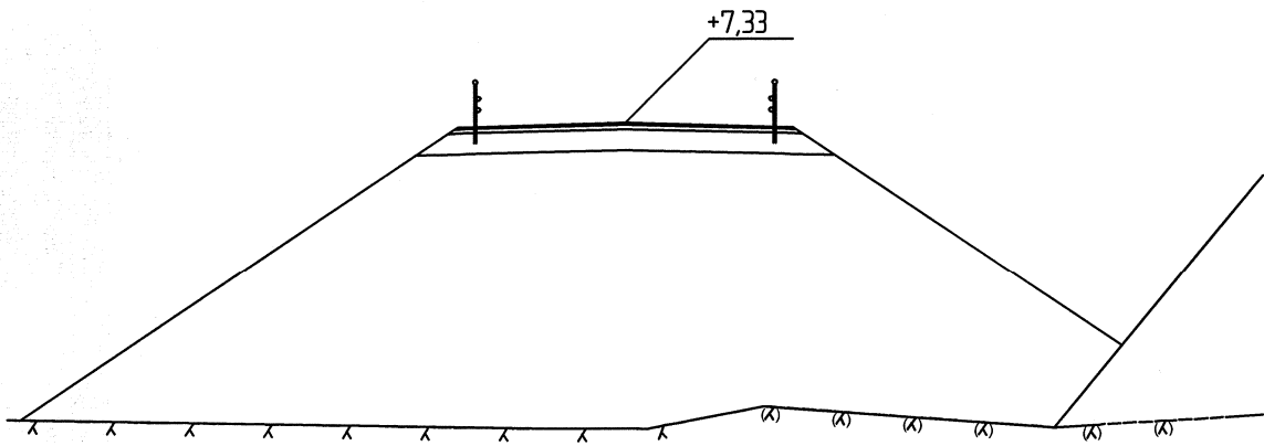
SEKTION 0/600
