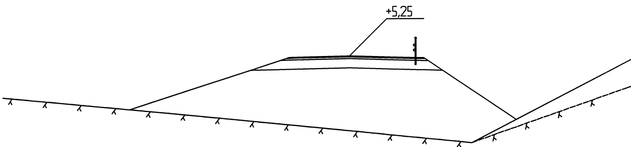
SEKTION 1/060
