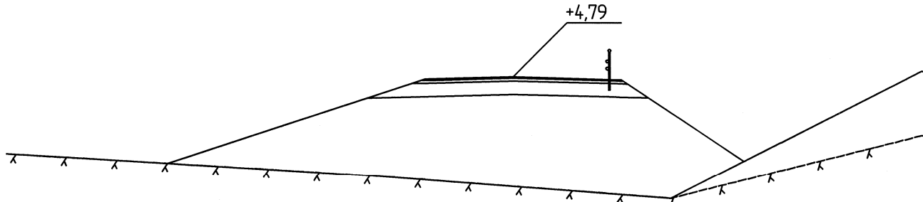
SEKTION 1/080
