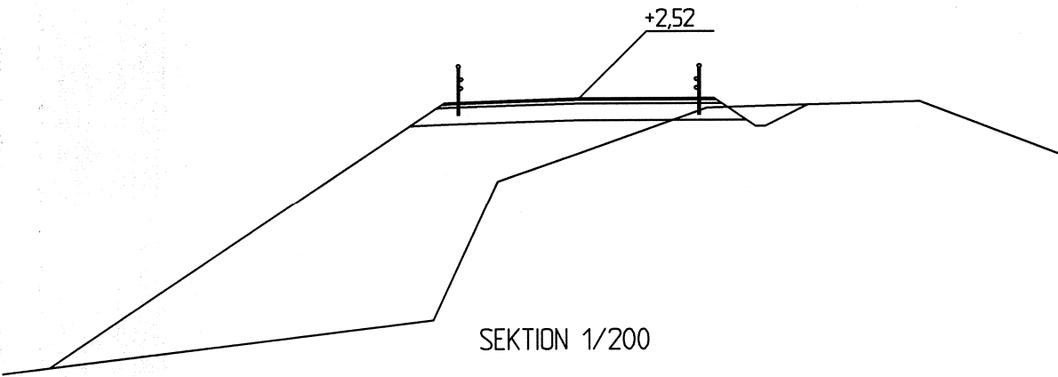
SEKTION 1/180
