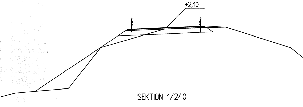
SEKTION 1/220
