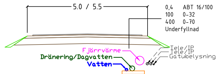
HAVTORNGRÄND TYPSEKTION 40m
