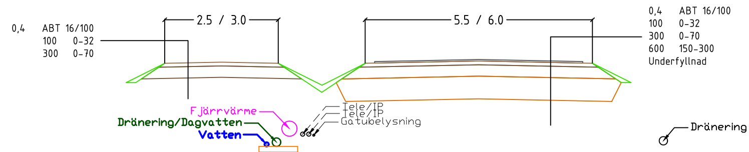
SANDBOLVÄGEN TYPSEKTION 360m
