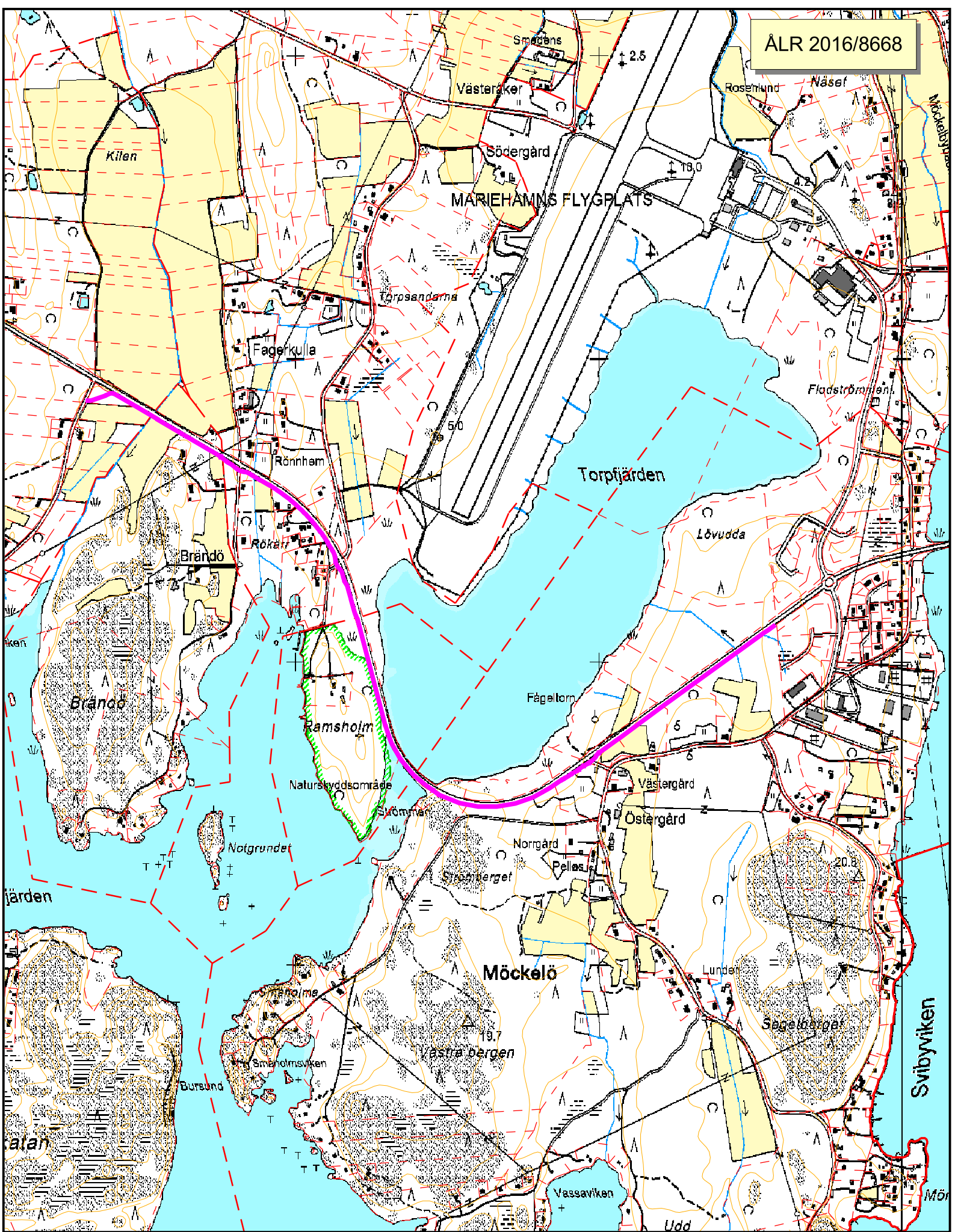
Vägplan för gc- väg intill landsväg 1, etapp 2, sektion 360- 3566
