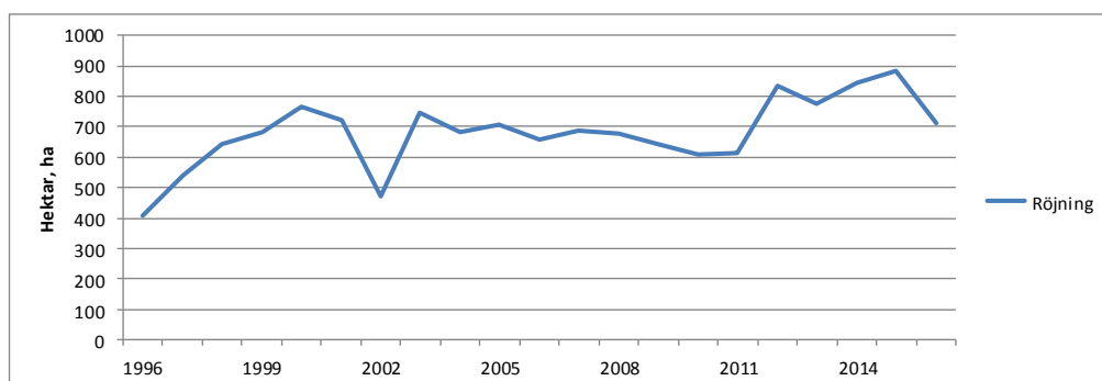
Figur 21. Plant- och ungsogsrøjning åren 1996-2016. (Källa: Ålands landskapsregering, skogsbruksbyrån).
