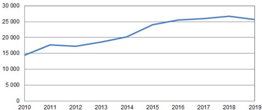
Antal storskarvsbon 2010–2019
