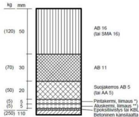
1a. Asfalttiberonipäällyste
