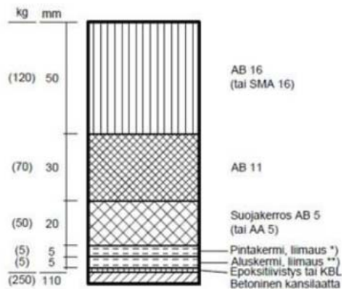
1a. Asfalttiberonipäällyste
