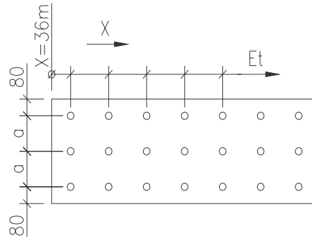
Blocket B2: mått riktning från stöd 2 till stöd 3
