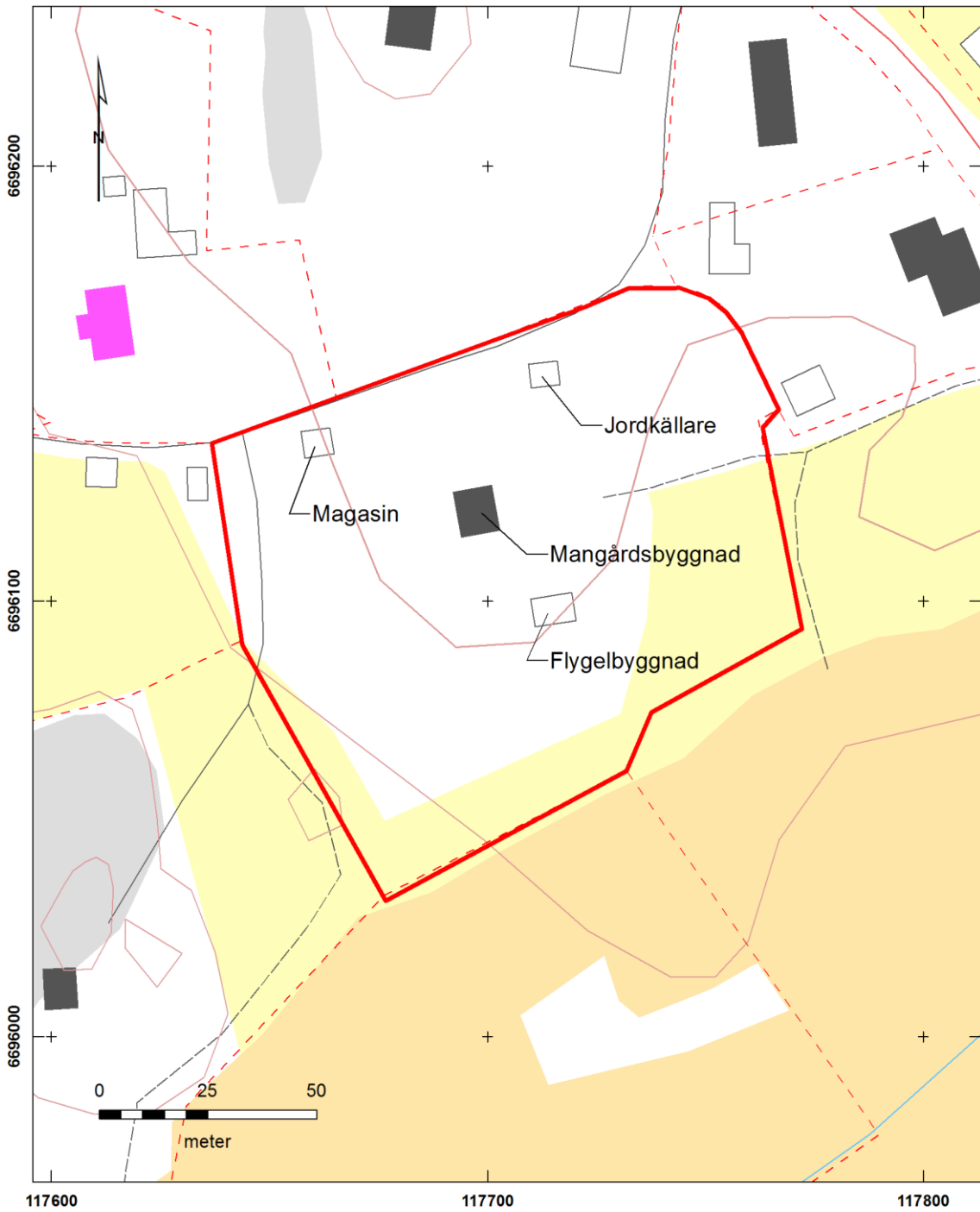
Figur 2: Översiktskarta, skala 1:1500
